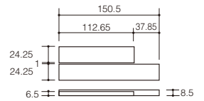
ECP-2515TNA タイル形状図(詳細)
