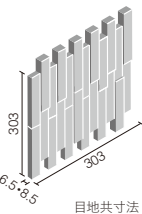
目地共寸法
