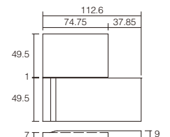
ECP-CTN シート形状図(詳細)
