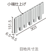
目地共寸法
