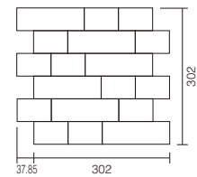
ECP-R シート形状図(詳細)
