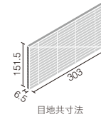
目地共寸法
