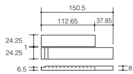
ECP-2515NB タイル形状図(詳細)
