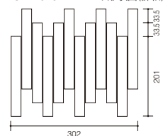
ECP-2520NET シート形状図(詳細)
