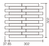
ECP-2515NET シート形状図(詳細)
