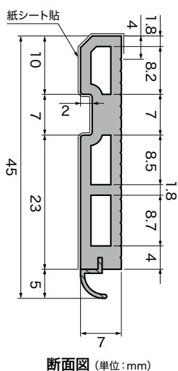
断面図 (単位:mm)
